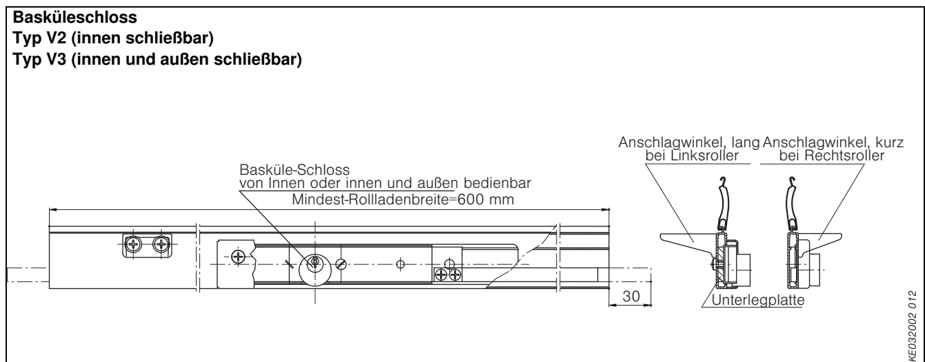
Abb. 82: Basküleschloss
