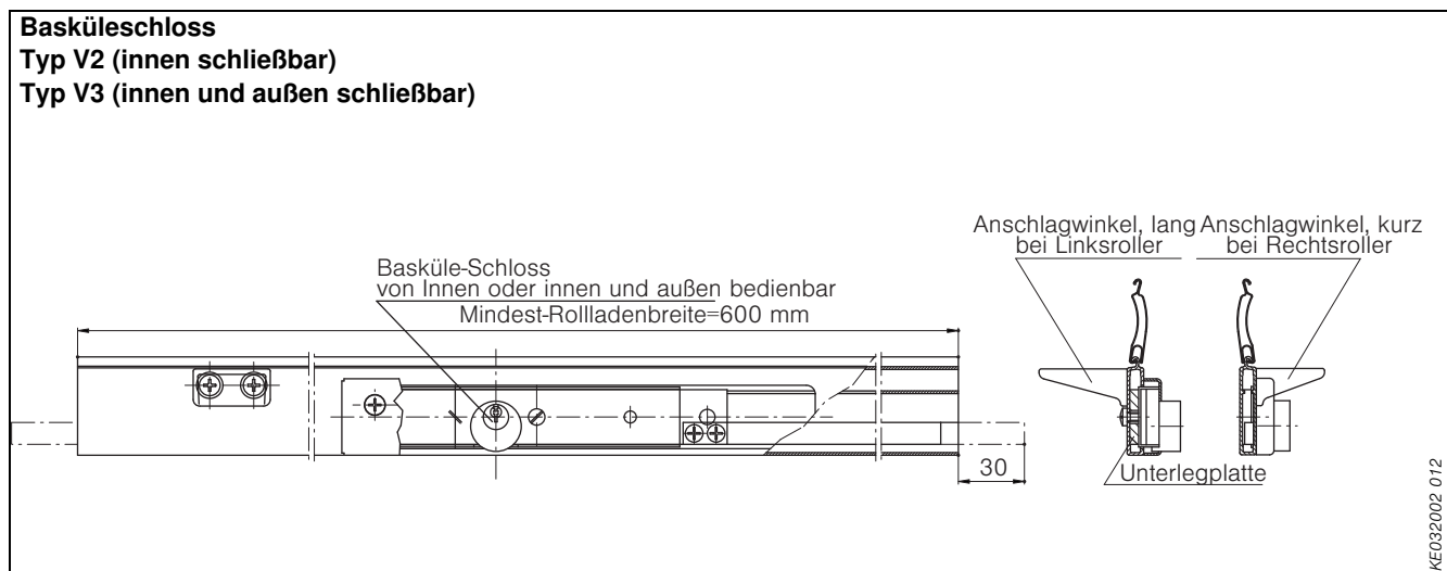
Abb. 82: Basküleschloss
