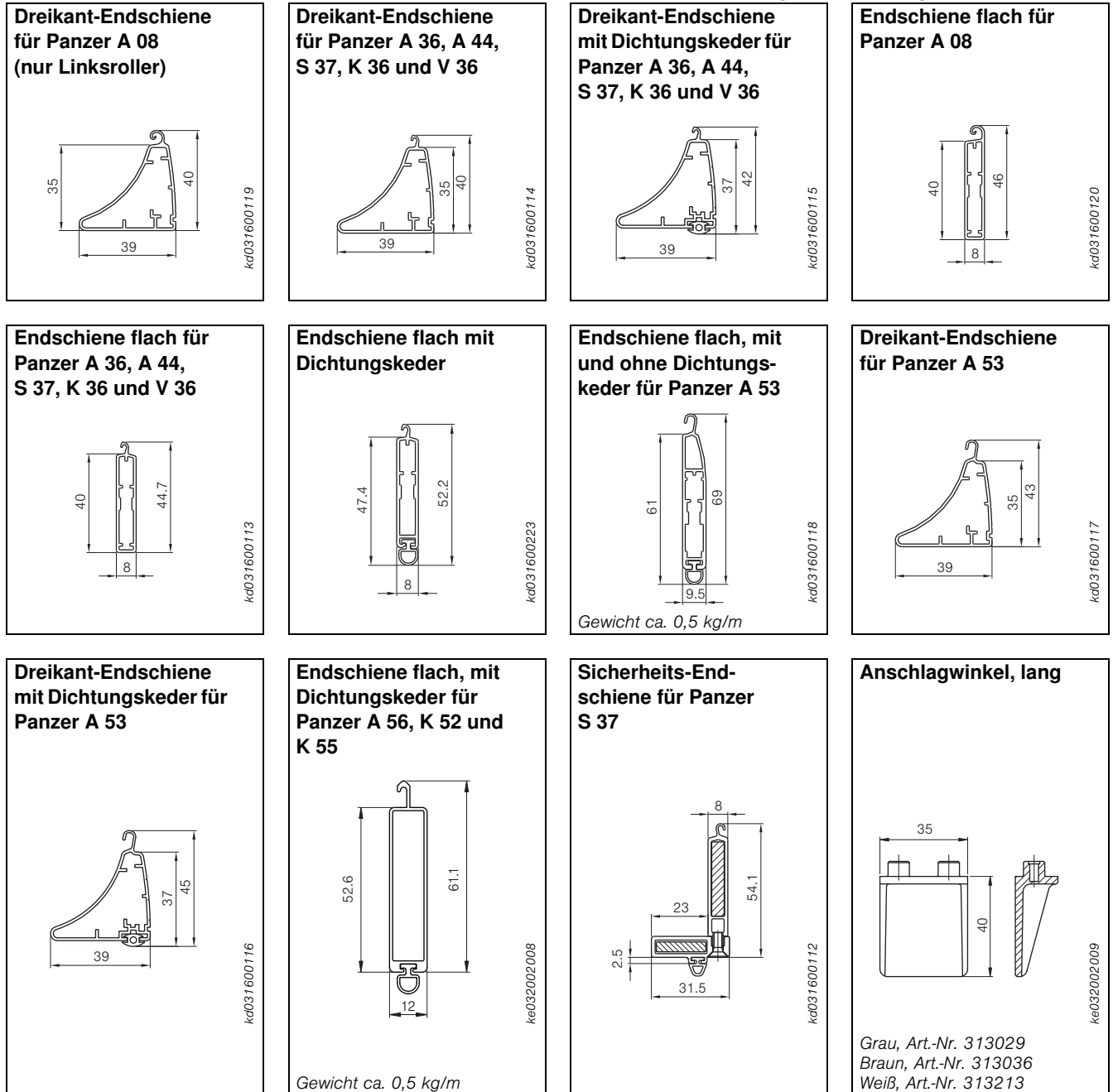
Abb. 80: Endschienen
