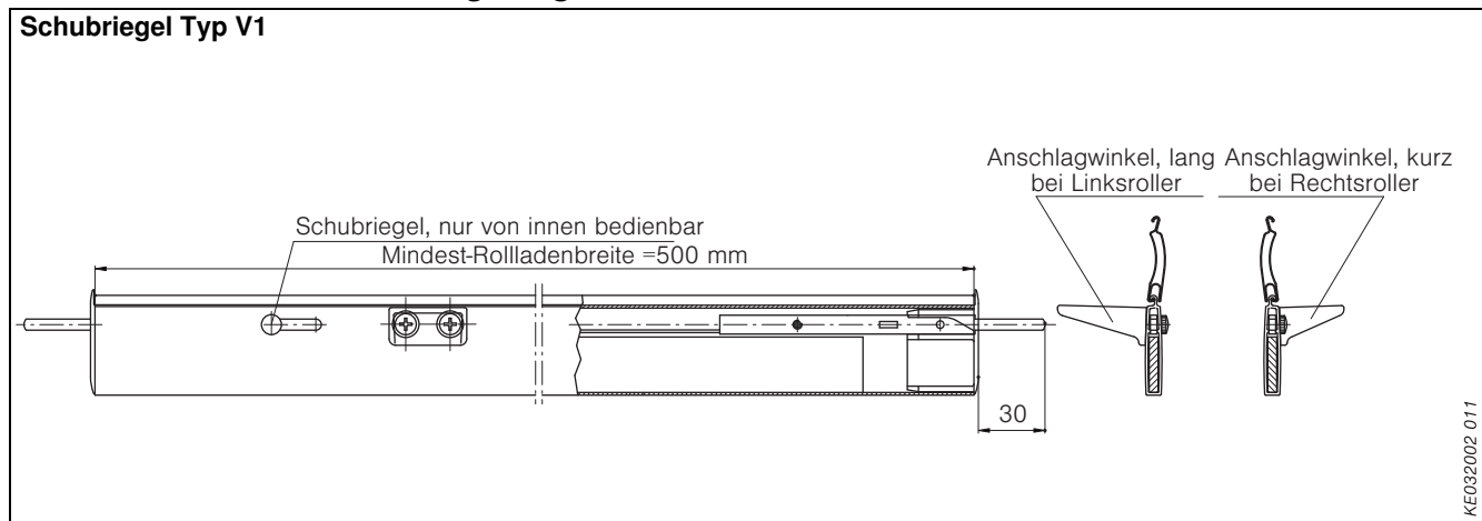
Abb. 81: Schubriegel
