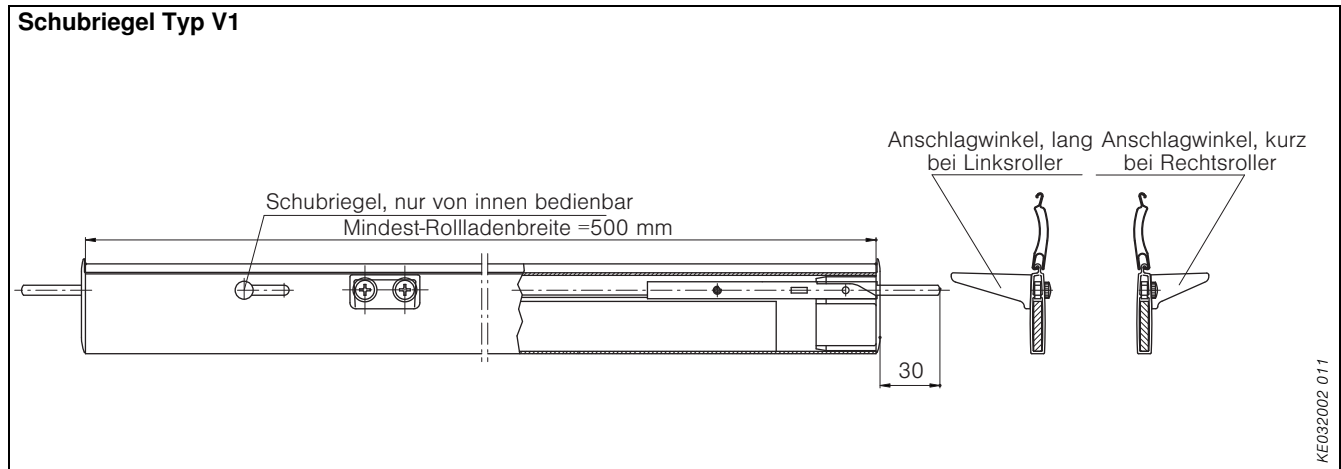
Abb. 81: Schubriegel
