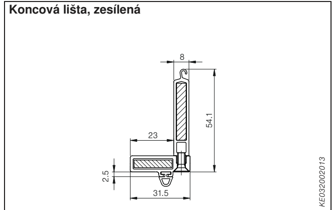
obr. 98: Koncová lišta
