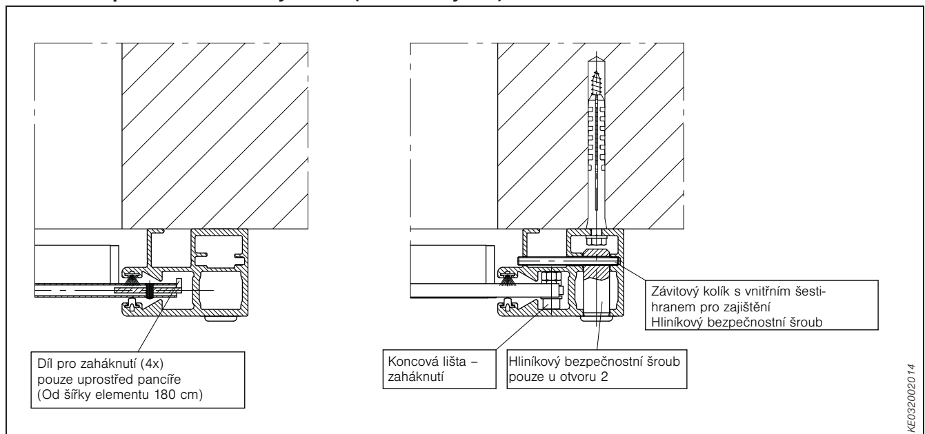
obr. 99: Zaháknutí pancíře a koncových lišt
