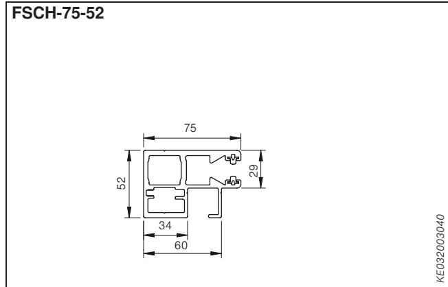
obr. 97: Standardní vodící lišta
